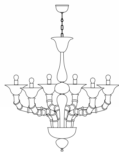
Art. F3946 / 6L. Dim. L 100 x 80 cm H 75 cm 6L E14 Max 40W
