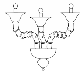
Art. F3946 / Apl. 3L. Dim. H 40 cm ø 58 cm P 37 cm 3L E14 Max 40W
