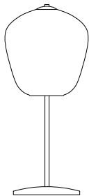
Art. AA187 / LG. Dim. H 61 cm Dim. vetro ø 28 cm Dim. base ø 25 cm 1L E27 Max 100W
