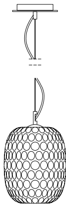
Art. AA153 / Sosp. Dim. H 30 / 130 cm Dim. Vetro ø 23 cm 1L E27 Max 60W
