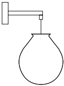
Art. AA188 / Apl. Dim. H 33 cm P 23 cm Dim. Vetro ø 20 cm 1L E14 Max 60W
