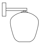
Art. AA187 / Apl. Dim. H 25 cm P 23 cm Dim. vetro ø 19 cm 1L E27 Max 60W
