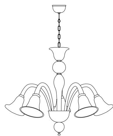
Art. F3930 5G. giù Dim. H 70 cm ø 80 cm 5L E14 Max 40W
