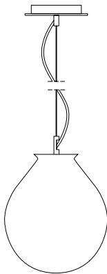
Art. AA188 / Sosp. G. Dim. H 35 / 130 cm Dim. Vetro ø 30 cm 1L E27 Max 100W
