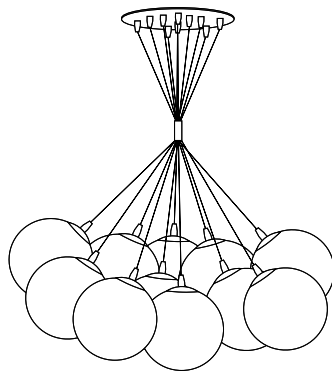
Art. AA178 / Sosp. 13L. Dim. 13 L ø 90 cm H 70 / 120 cm 13 L E27 Max 60W Dim. Sfera ø 20 cm
