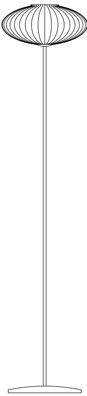
Art. AA151 / LT. Dim. H 165 cm Dim. Vetro ø 30 cm Dim. Base ø 30 cm 1L E27 Max 60W
