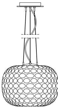
Art. AA152 / Sosp. Dim. H 25 / 130 cm Dim. vetro ø 32 cm 1L E27 Max 100W
