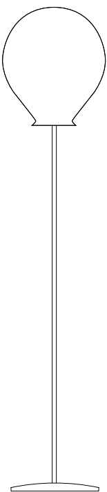
Art. AA188 / LT. Dim. H 180 cm Dim. Vetro ø 30 cm Dim. Base ø 30 cm 1L E27 Max 100W
