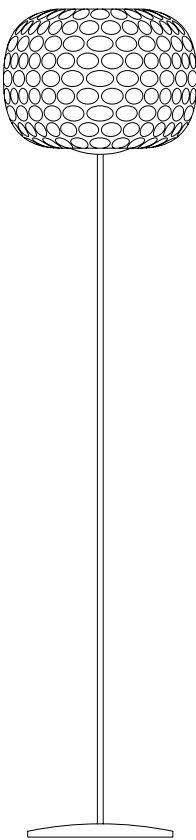
Art. AA152 / LT. Dim. H 170 cm Dim. vetro ø 32 cm Dim. base ø 30 cm 1L E27 Max 100W
