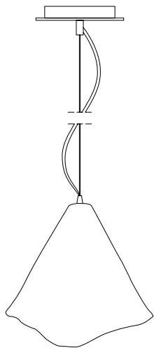
Art. AA189 / Sosp. G. Dim. H 44 / 130 cm Dim. Vetro ø 46 cm 1L E27 Max 100W
