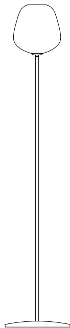
Art. AA187 / LT. Mini Dim. H 167 cm Dim. vetro ø 19 cm Dim. base ø 30 cm 1L E27 Max 60W
