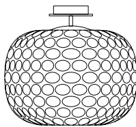
Art. AA152 / PL. Dim. H 31 cm Dim. Vetro ø 32 cm 1L E27 Max 100W
