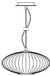
Art. AA151 / Sosp. Dim. H 16 / 130 cm Dim. Vetro ø 30 cm 1L E27 Max 60W
