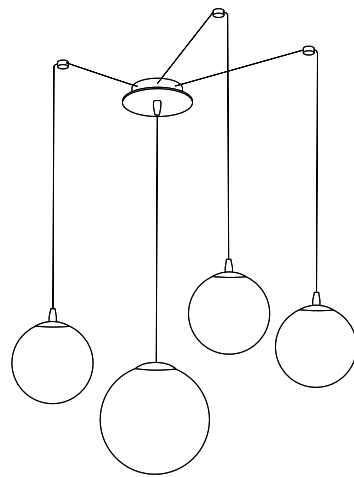
Art. AA178 / Sosp. Decentrata Dim. 4L H 36 / 130 cm regolabili ø 90 Dim. 1 Sfera ø 30 e 3 Sfere ø 20 cm 4L E27 Max 60W
