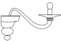
Art. F3327 / A1 Mod. Dim. H 20 cm P 25 cm ø 15 cm 1L E14 Max 40W
