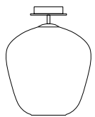
Art. AA187 / PL. G. Dim. H 38 cm Dim. vetro ø 28 cm 1L E14 Max 100W
