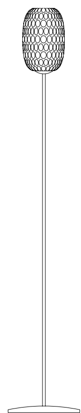
Art. AA154 / LT. Dim. H 167 cm Dim. Vetro ø 14 cm Dim. Base ø 30 cm 1L E27 Max 60W
