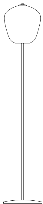
Art. AA187 / LT. Dim. H 160 cm Dim. vetro ø 28 cm Dim. base ø 30 cm 1L E27 Max 100W
