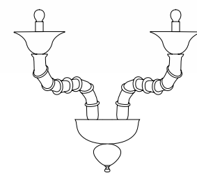
Art. F3946 / Apl. 2L. Dim. H 35 cm ø 45 cm P 28 cm 2L E14 Max 40W
