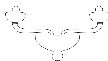
Art. F3944 / A2 L Dim. L 40 cm H 30 cm P 28 cm 2L E14 Max 40W
