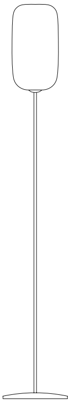
Art. AA179 / LT. Dim. ø 30 cm H 187 cm Dim. Base ø 30 cm 1L E27 Max 100W
