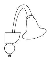
Art. F3930 Apl. 1 Dim. H 28 cm ø 15 cm P 29 cm 1L E14 Max 40W
