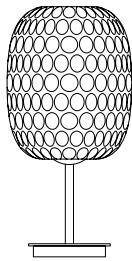
Art. AA153 / LG. Dim. H 50 cm Dim. Vetro ø 23 cm Dim. Base ø 22 cm 1L E27 Max 100W
