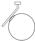
Art. AA178 / Apl. / Sosp. Asta Dim. H 50 cm L 36 cm Dim. Sfera ø 30 cm 1L E27 Max 60W
