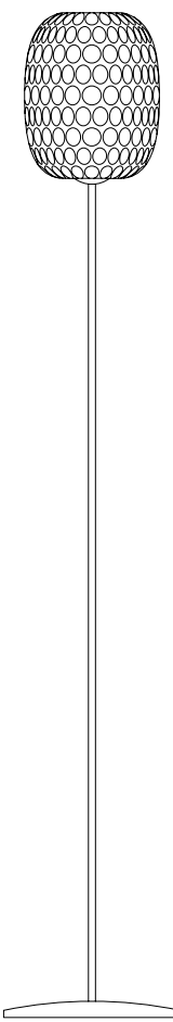
Art. AA153 / LT. Dim. H 175 cm Dim. Vetro ø 23 cm Dim. Base ø 30 cm 1L E27 Max 100W
